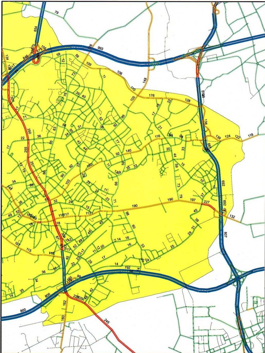
Verkehrsbelastungen für die Variante 1, Werktagsverkehr 2020 in 100 Kfz/24h Ausschnitt Bottrop
