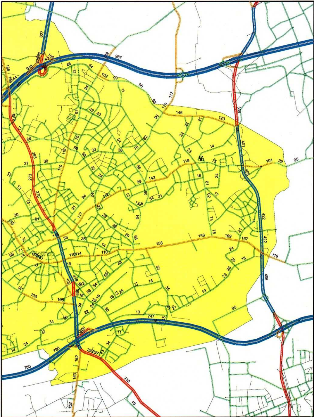
Verkehrsbelastungen für den Prognose-0-Fall, Werktagsverkehr 2020 in 100 Kfz/24h Ausschnitt Bottrop
